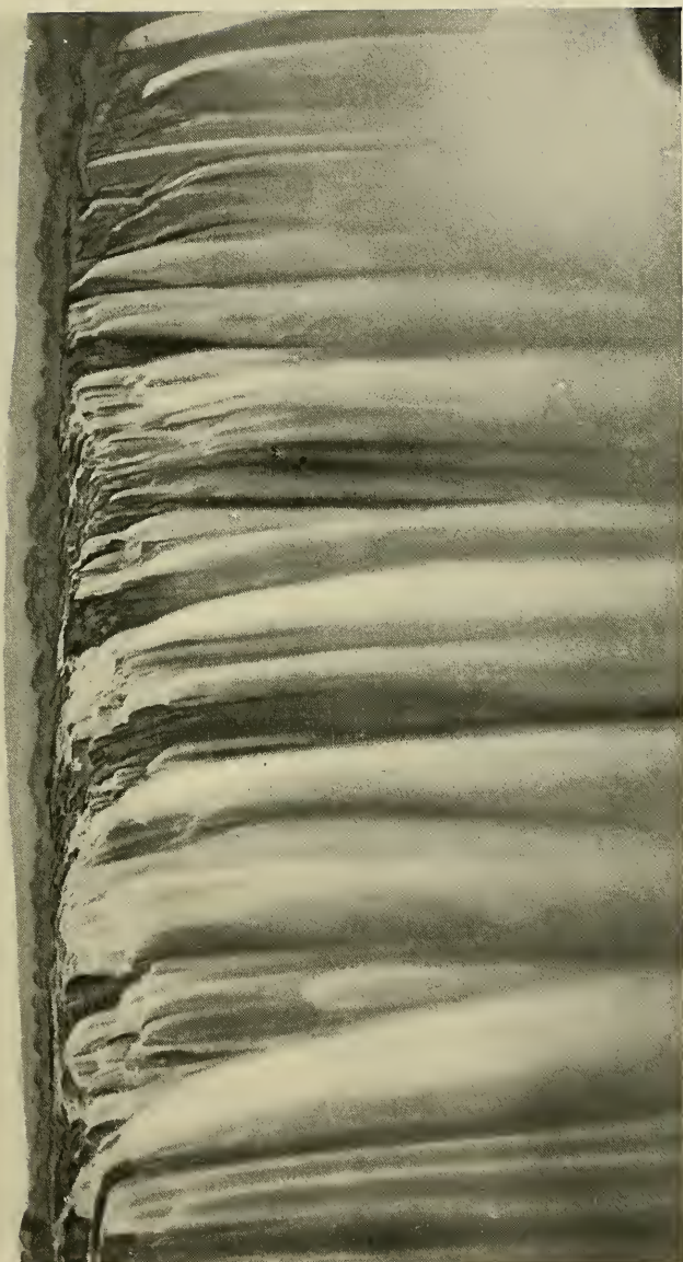
FALLS OF THE ZAMBESI.
